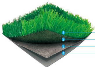
人造草结构图
